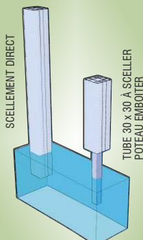
POTEAU À SCELLER
