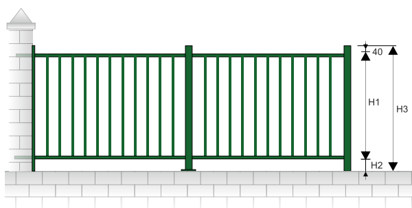
Clôture Barreadée City 2 traverses sans fer de lance
