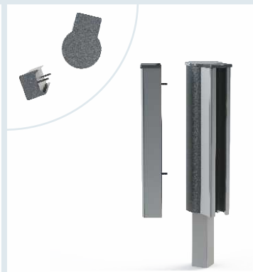
Poteau d'angle avec tube 30x30 à sceller
